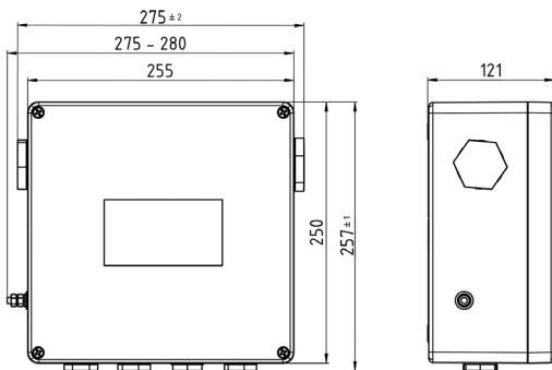
Габаритные размеры
